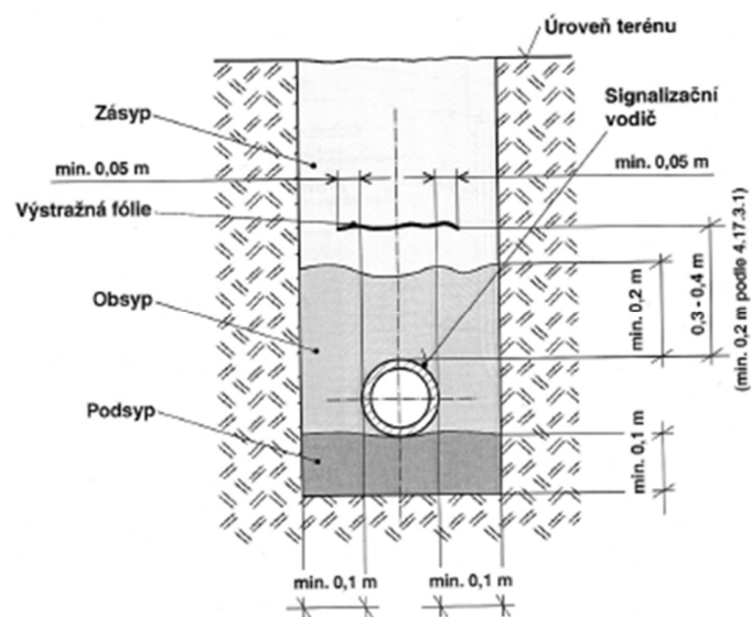
Příklad uložení trubek v otevřeném výkopu Obr.č.8
